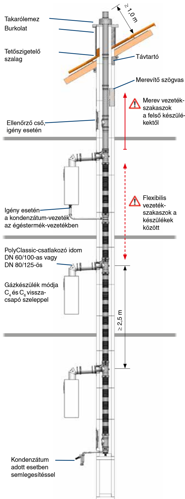
Többrákötésű PolyCase tipikus felépítése
